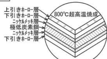
ホーロー鋼板の断面構造図 ※下引き、上引きを施したデュアルコートであること
